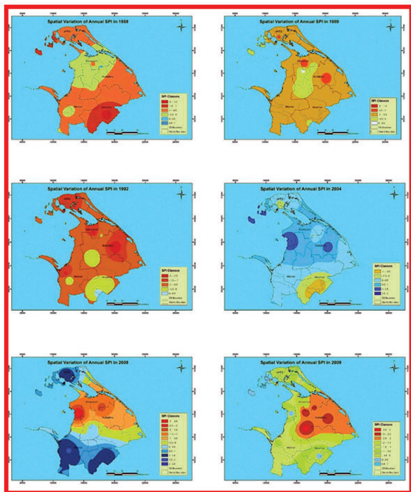
படம் 12.4 கடந்த காலங்களில் வரட்சியின் இடம் சார்ந்த பாங்கு - நியமமாக்கப்பட்ட வீழ்ச்சியின் குறிகாட்டி அடிப்படையினானது
