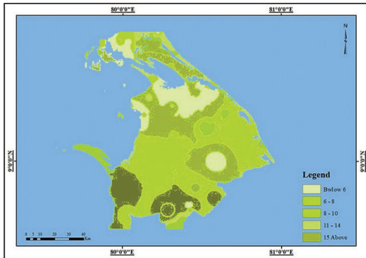
படம் 12.3 வடக்கு மாகாணத்தில் 2012 முதல் 2022 வரையான காலப்பகுதியில் நிகழ்ந்த வறட்சி நிகழ்வுகளின் எண்ணிக்கையின் இடம்சார்ந்த பரம்பல்
