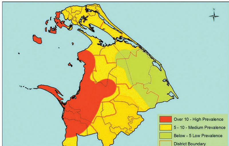
படம். 12.5 வடக்கு மாகாணத்தின் வரட்சியின் நிகழ்வு எண்ணிக்கையின் அடிப்படையில் அதிகளவு, நடுத்தர மற்றும் குறைந்த வரட்சி நிகழ்வுப் பிரதேசங்கள். மாகாணத்தின் மேற்குப் பகுதிகள் அதிகளவு வரட்சியையும் கிழக்குப் பகுதிகள் குறைந்த வரட்சியையும் கொண்டிருக்கின்றன.
