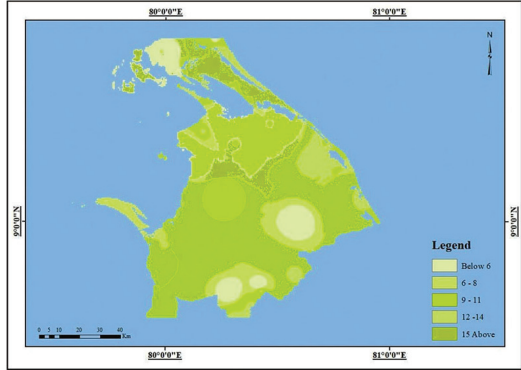
படம் 12.2 வடக்கு மாகாணத்தில் 2002 முதல் 2012 வரையான காலப்பகுதியில் நிகழ்ந்த வறட்சி நிகழ்வுகளின் எண்ணிக்கையின் இடம்சார்ந்த பரம்பல்
